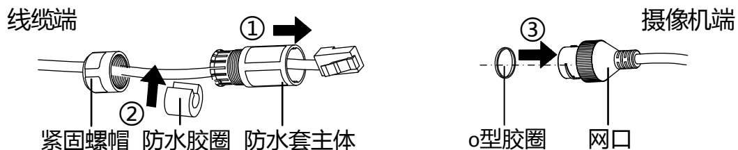
图1-6 安装网线
