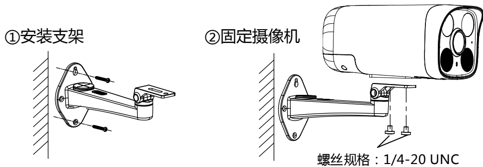
图1-1 安装摄像机
