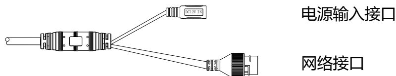
图1-2 线缆说明
