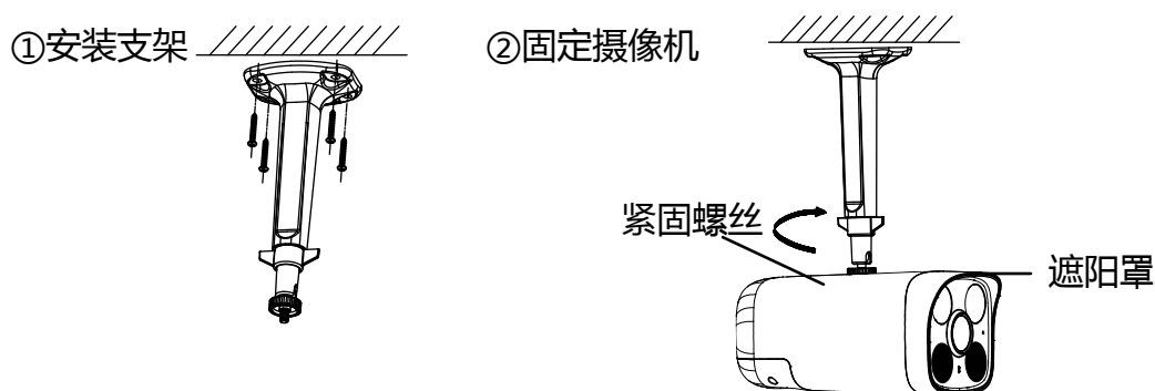
图1-4 安装摄像机
