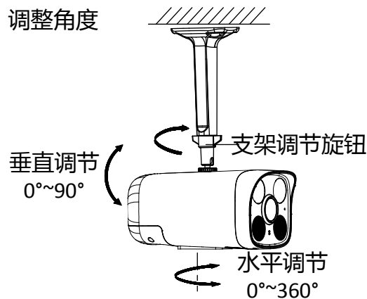
图1-5 调整角度
